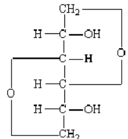
Isosorbid
