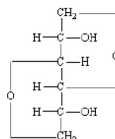
Isosorbitid
