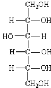
Sorbitol
