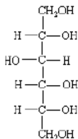
Sorbitol
