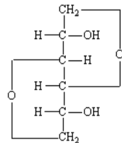
Isosorbitid
