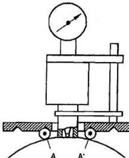
Hình C.1 - Thử nghiệm trên các bề mặt có bán kính cong lớn
