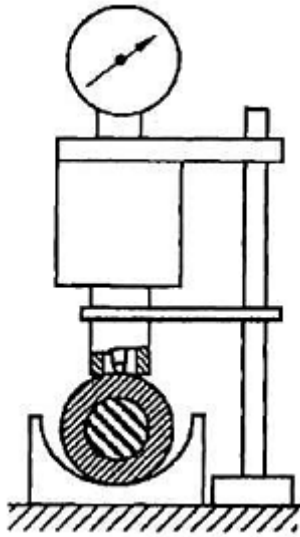
Hình C.2a - Mảnh thử nghiệm trong rãnh
